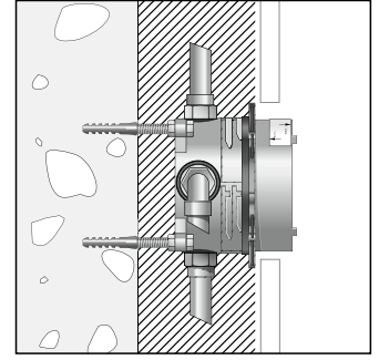
Duvarın tam önüne uygulanabilen tesisat ve M 10 askı civatalı ayrıcılar
