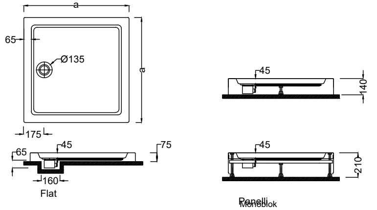
Monoblok h:14 cm
